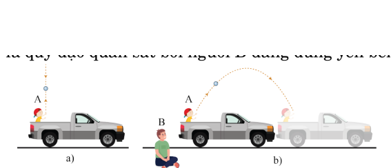
(a) Quỹ đạo thẳng (quan sát bởi người A trên xe) (b) Quỹ đạo parabol (quan sát bởi người B đứng bên đường)
